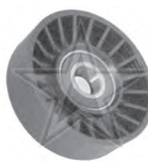
8033 A=25 DI=17 DE=82 mm
